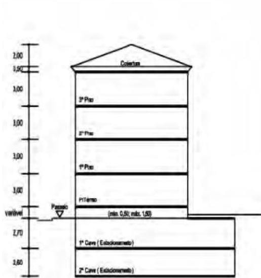
Edifício Habitacional
